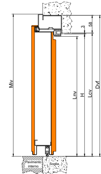
SEZIONE VERTICALE VERTICAL SECTION
