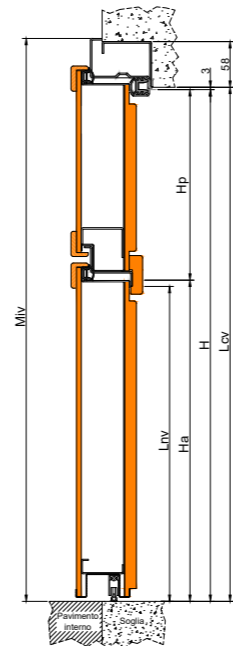
SEZIONE VERTICALE VERTICAL SECTION
