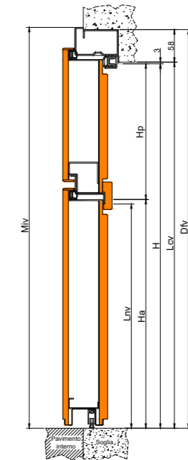
SEZIONE VERTICALE VERTICAL SECTION
