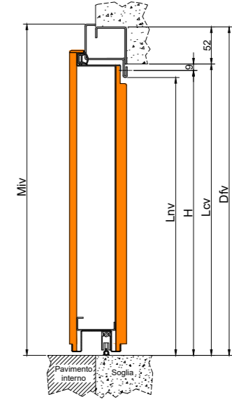
SEZIONE VERTICALE VERTICAL SECTION
