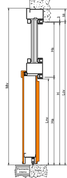
SEZIONE VERTICALE VERTICAL SECTION
