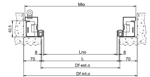
SEZIONE ORIZZONTALE HORIZONTAL SECTION
