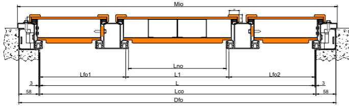
SEZIONE ORIZZONTALE HORIZONTAL SECTION
