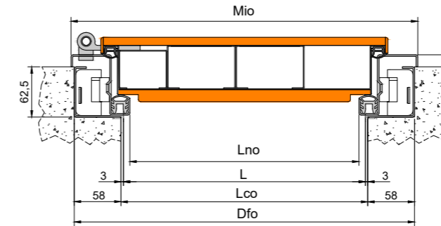
SEZIONE ORIZZONTALE HORIZONTAL SECTION
