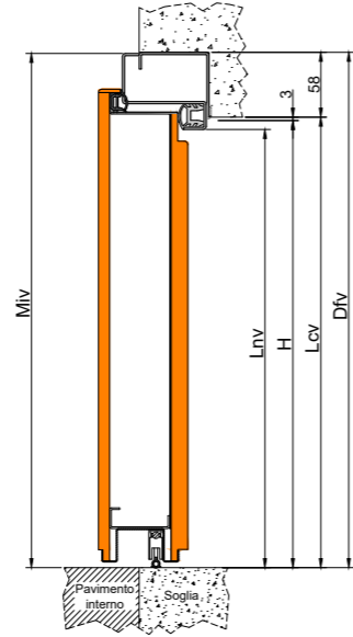
SEZIONE VERTICALE VERTICAL SECTION
