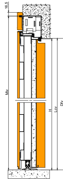
SEZIONE VERTICALE VERTICAL SECTION
