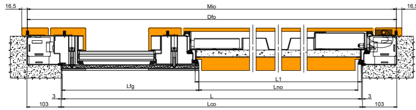
SEZIONE ORIZZONTALE HORIZONTAL SECTION
