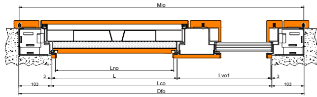
SEZIONE ORIZZONTALE HORIZONTAL SECTION
