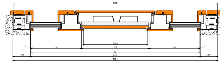
SEZIONE ORIZZONTALE HORIZONTAL SECTION
