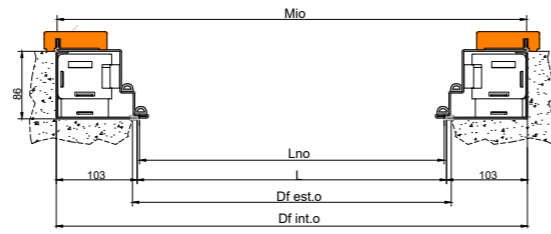
SEZIONE ORIZZONTALE HORIZONTAL SECTION
