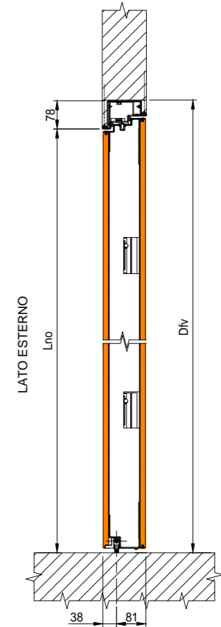
SEZIONE VERTICALE VERTICAL SECTION
