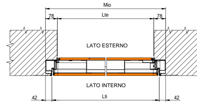
SEZIONE ORIZZONTALE HORIZONTAL SECTION
