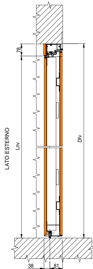
RASO MURO ESTERNO E INTERNO
